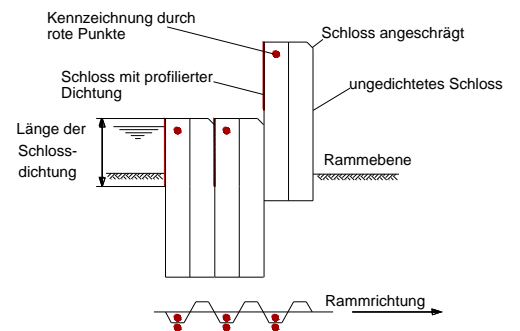
Schloss mit profilierter Dichtung Mittelschloss mit injizierter Dichtung
