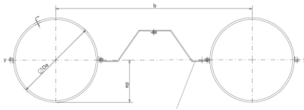
Rohrspundwand mit Hoesch 1907 DB als Zwischentafel
